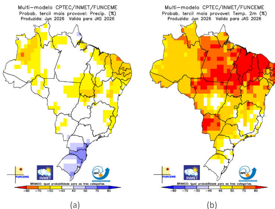
Figura 3: Previsão climática sazonal por tercil (categorias abaixo da faixa normal, dentro da faixa normal e acima da faixa normal), gerada pelo método objetivo (CPTEC/INPE, INMET e FUNCEME). As áreas em branco indicam igual probabilidade para as três categorias. (a) precipitação; (b) temperatura.
